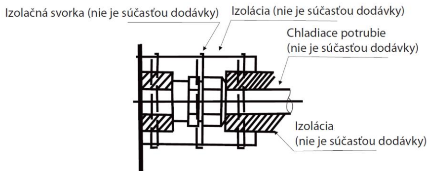
Postup izolácie potrubia
